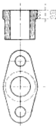
Fig. 6. Wie Fig. 5, nach vereinfacht, in der Praxis zulässiger Art gezeichnet. Die strichpunktierte Ergänzung dient zur Klarstellung des Längsschnittes.
