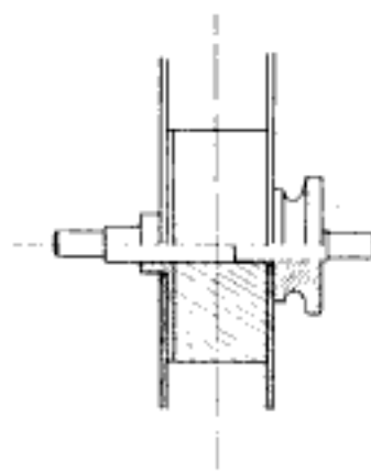
Fig. 8. Die Achse ist in Ansicht, Scheibe u. s. w. dagegen im Schnitt und unsichtbare Linien, wo möglich, nicht gezeichnet.
