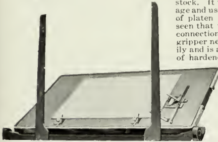
Fig. 1. Platen Open
