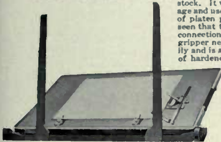
Fig. 1. Platen Open
