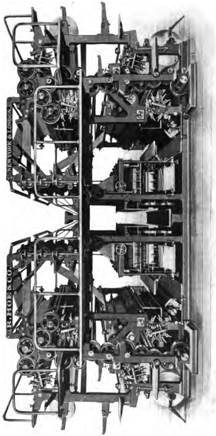
OCTUPLE PRESS
